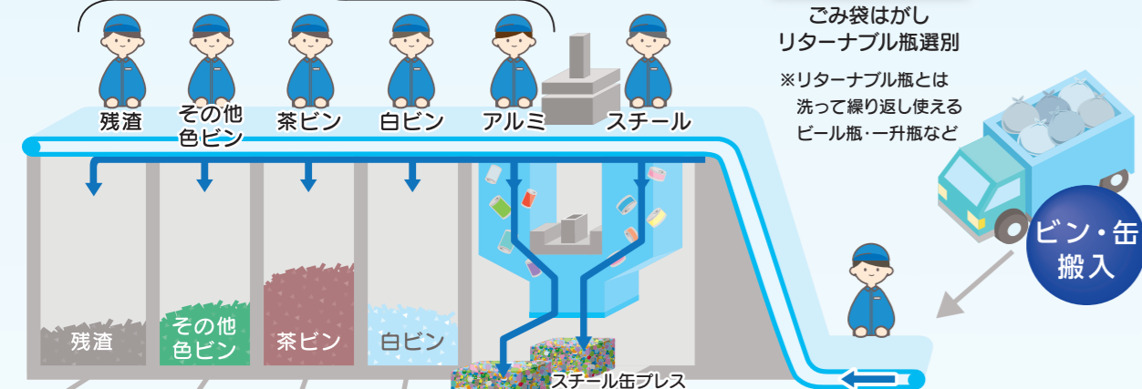
手選別ライン 磁力選別(スチール回収) ごみ袋はがし
